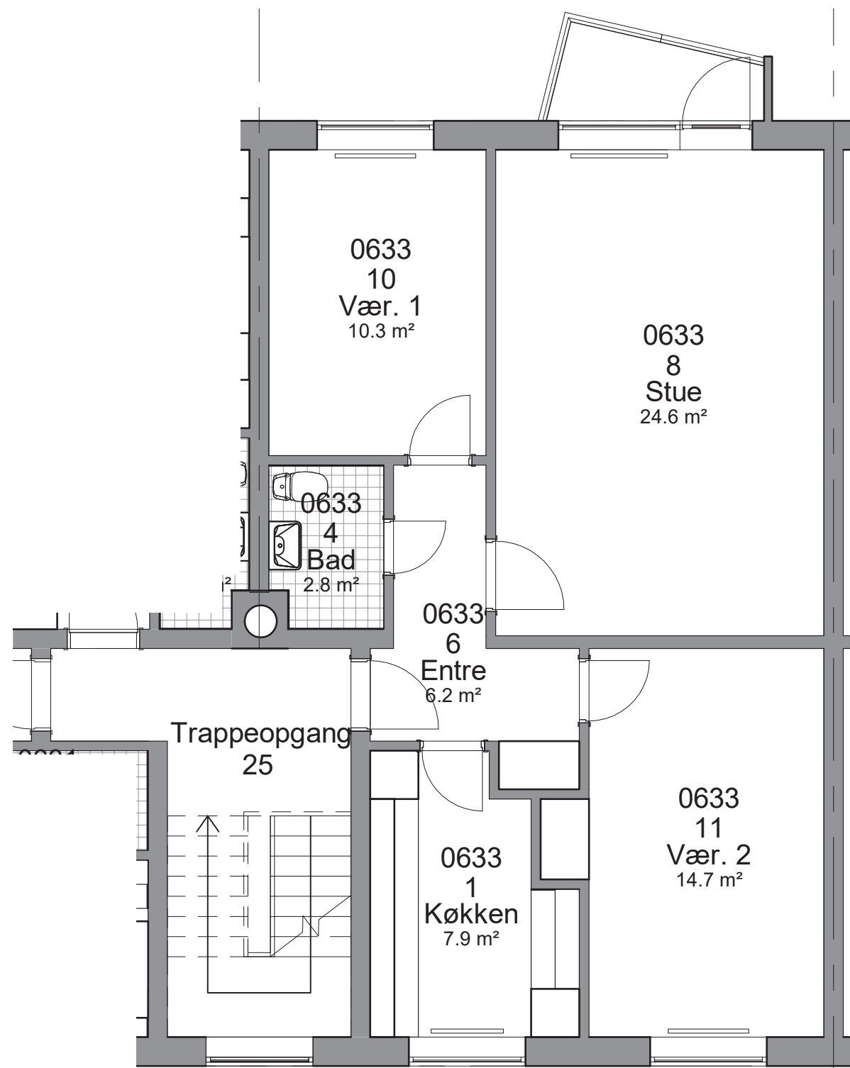
EKSISTERENDE FORHOLD 83 M 2 3-VÆRELSES BOLIG
