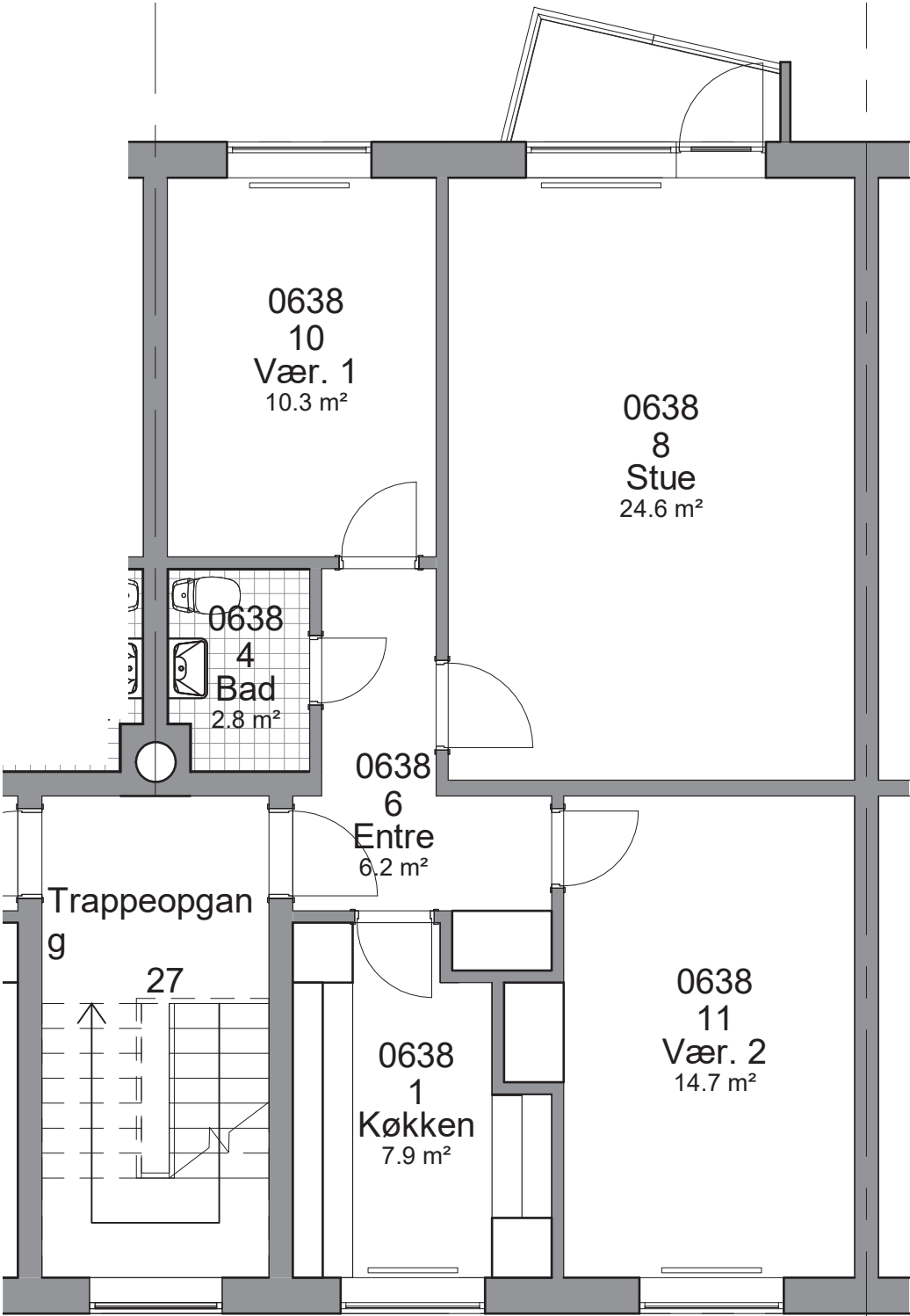
EKSISTERENDE FORHOLD 84 M² 3-VÆRELSES BOLIG
