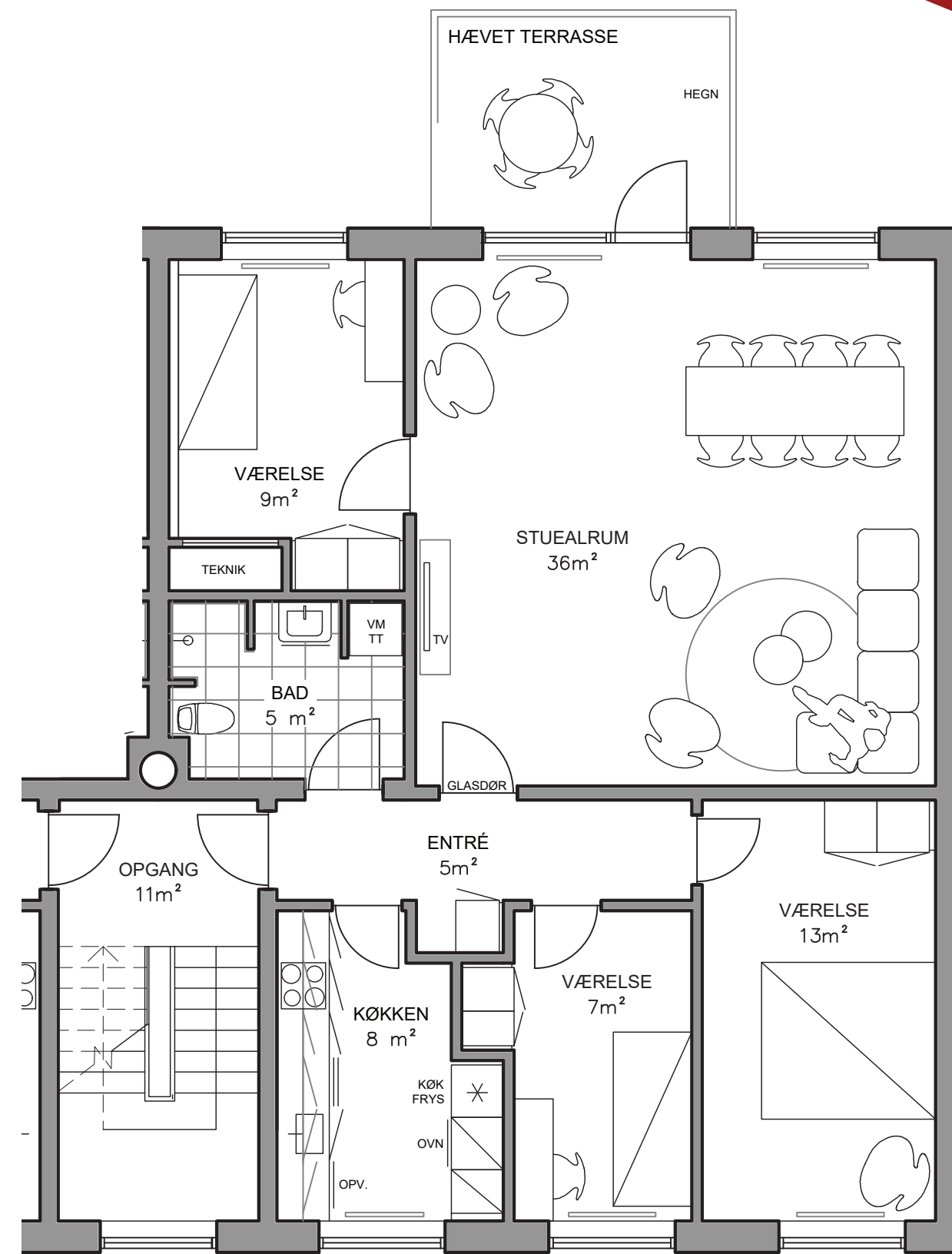
FREMTIDIG FORHOLD 109 M 2 4-VÆRELSES BOLIG
