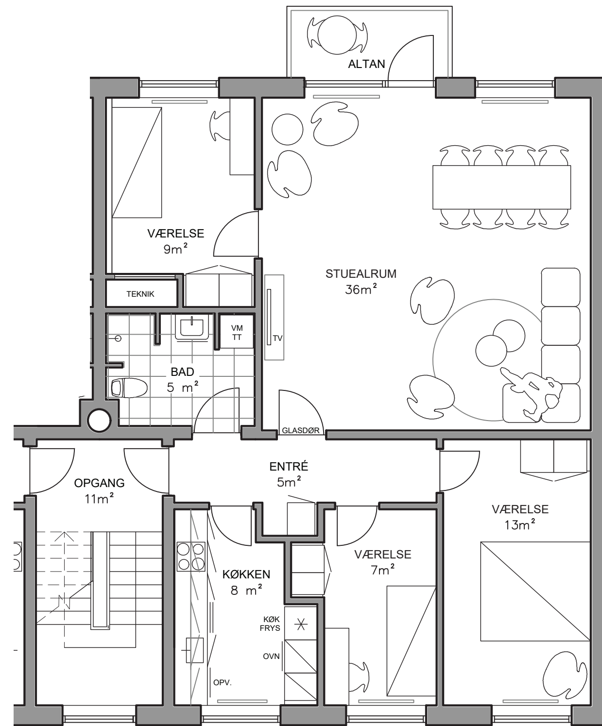
FREMTIDIG FORHOLD 109 M 2 4-VÆRELSES BOLIG
