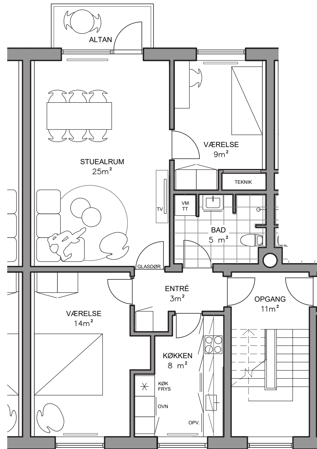
FREMTIDIG FORHOLD 84 M² 3-VÆRELSES BOLIG
